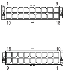
SSI_2X9P
