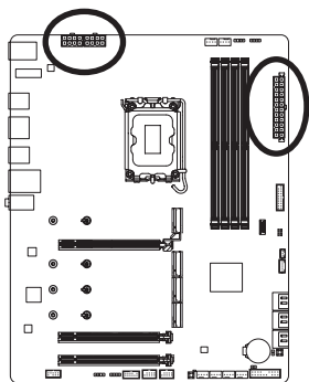
ATX_12V_2X4_1 / ATX_12V_2X4_2
