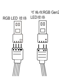
RGB LED燈條插頭接腳：
