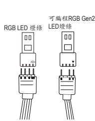
RGB LED燈條插頭接腳：
