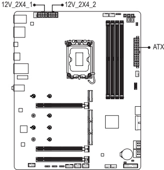
12V_2X4_1/12V_2X4_2:
