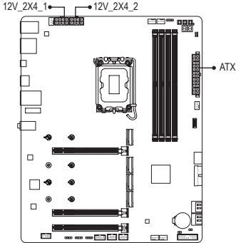
12V_2X4_1/12V_2X4_2:
