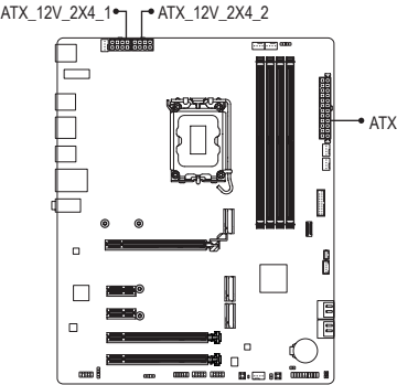
ATX_12V_2X4_1/2:
