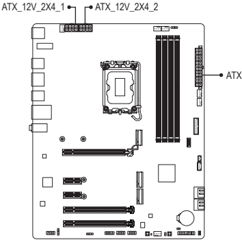
ATX_12V_2X4_1/2:
