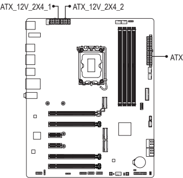
ATX_12V_2X4_1/2:
