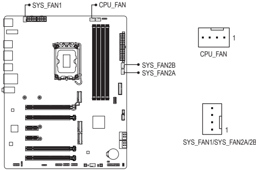
CPU_FAN/SYS_FAN1/SYS_FAN2A :
