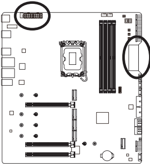
ATX_12V_2X4_1/ATX_12V_2X4_2
