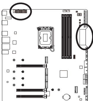
ATX_12V_2X4_1/ATX_12V_2X4_2
