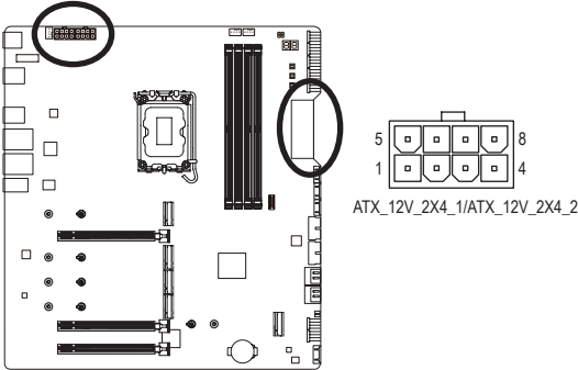
ATX_12V_2X4_1/ATX_12V_2X4_2:
