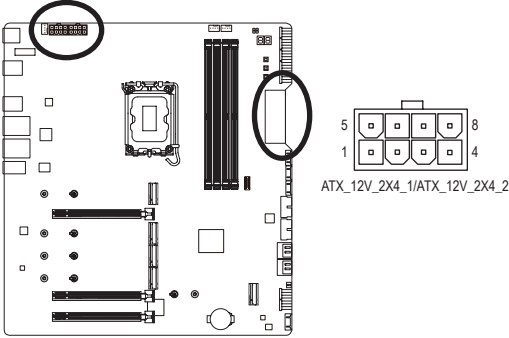
ATX_12V_2X4_1/ATX_12V_2X4_2 :
