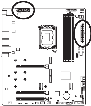
ATX_12V_2X4_1/ATX_12V_2X4_2
