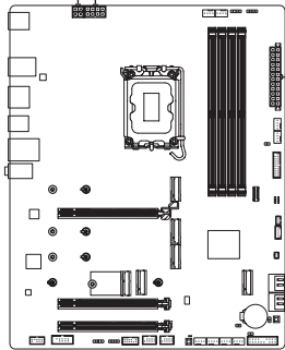
ATX_12V_2X2
