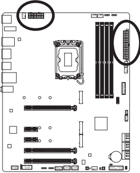
ATX_12V_2X2
