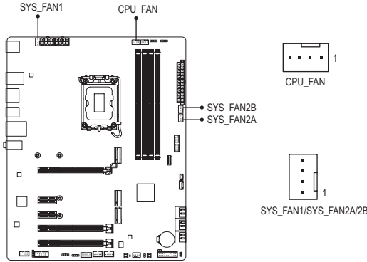
CPU_FAN/SYS_FAN1/2A :
