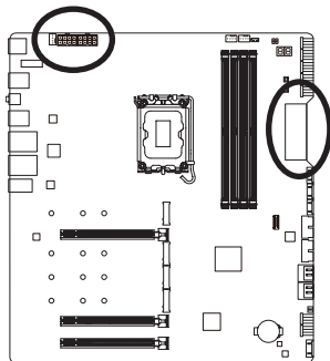
ATX_12V_2X4_1/ATX_12V_2X4_2
