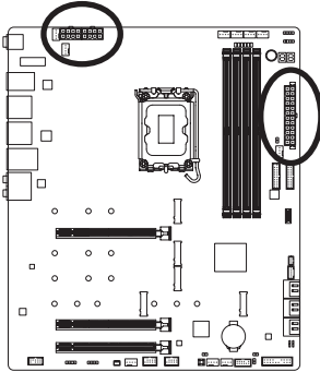
ATX_12V_2X4_1/ATX_12V_2X4_2
