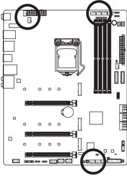
SYS_FAN3/SYS_FAN4
