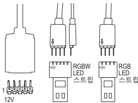
LED_C2
