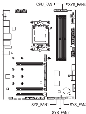
CPU_FAN/SYS_FAN4
