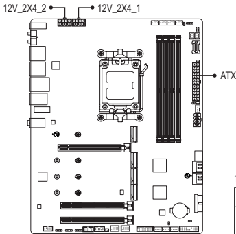
12V_2X4_1/12V_2X4_2 :
