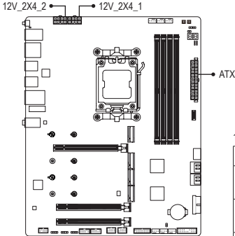
12V_2X4_1/12V_2X4_2:
