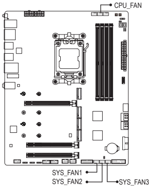
SYS_FAN1/SYS_FAN2/SYS_FAN3
