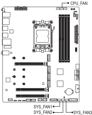
SYS_FAN1/SYS_FAN2/SYS_FAN3
