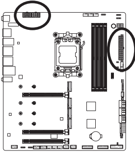
ATX_12V/ATX_12V1:
