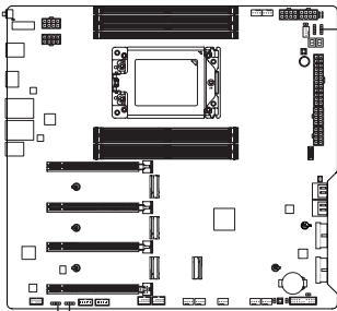
ARGB_V2_3/ARGB_V2_1
