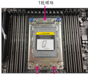
步驟一： 3號螺絲 2號螺絲
