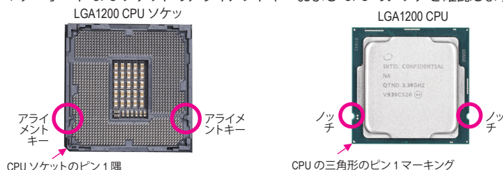
CPU ソケットのピン1隅
