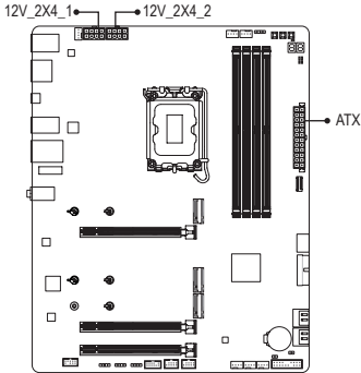
12V_2X4_1/12V_2X4_2:
