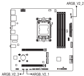
ARGB_V2_1/ARGB_V2_3
