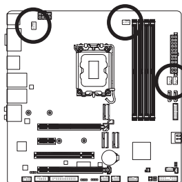
SYS_FAN1
