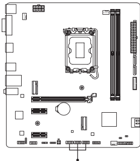
F_USB1/F_USB2/F_USB3
