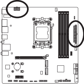
ATX_12V:
