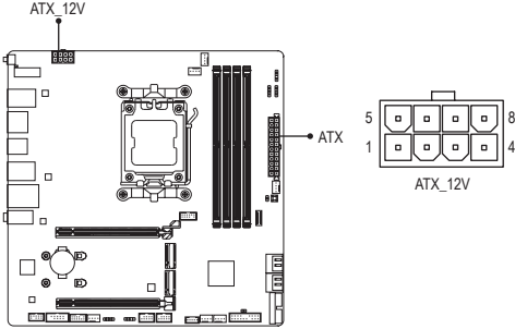
ATX_12V :
