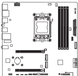
CLR_CMOS
