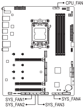
SYS_FAN1/SYS_FAN2/ SYS_FAN3/SYS_FAN4
