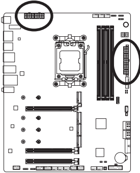
ATX_12V/ATX_12V1:
