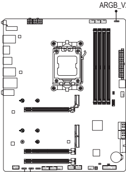
ARGB_V2_3 ARGB_V2_1
