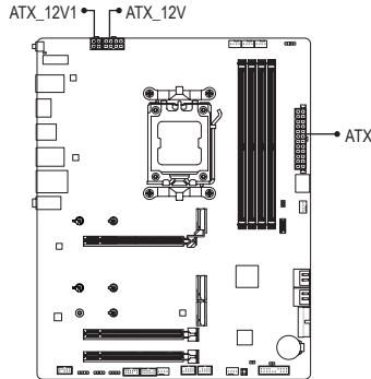
ATX_12V:
