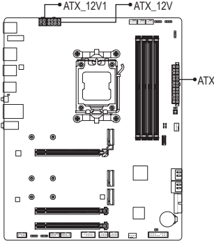
ATX_12V:
