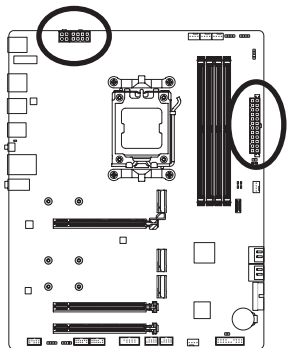
ATX_12V:
