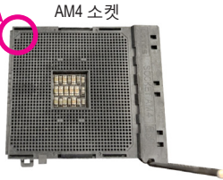
AM4 소켓
