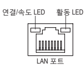
연결/속도 LED:
