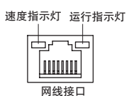
速度指示灯:
