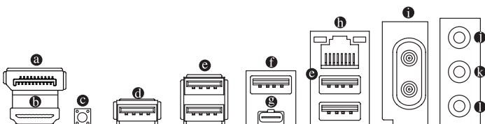
Вид сзади-А
