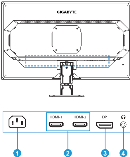
1 Wechselspannungseingang
