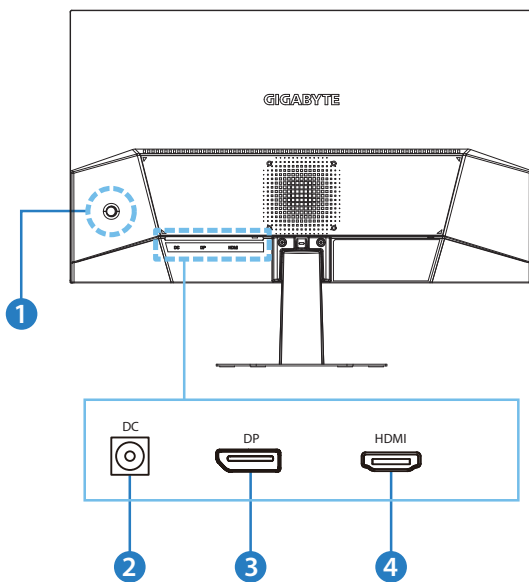
1 コントロールボタン
