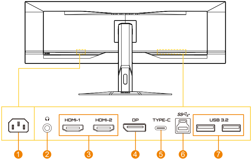
1 שקע AC IN 2 שקע לאוזניות 3 יציאות HDMI (x2) 4 DisplayPort 5 יציאת USB Type-C 6 יציאת USB להעלאה 7 יציאות USB 3.2 (x2)
